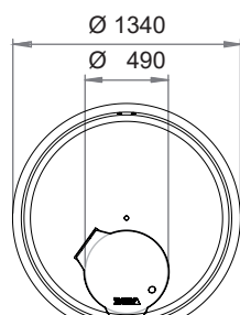
Horní pohled
