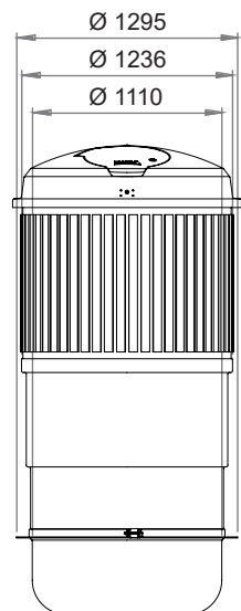
Čelní pohled
