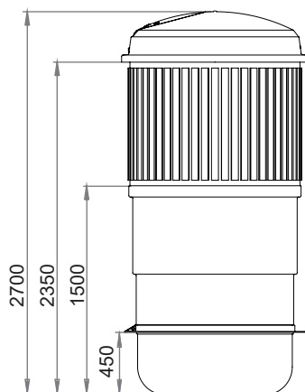
Boční pohled
